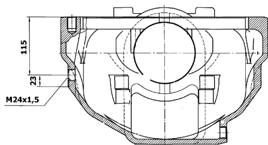
Рис. 2. Картер ведущего моста
